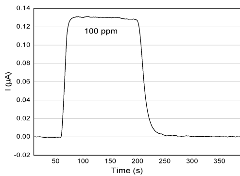
传感器灵敏度及响应恢复特性
